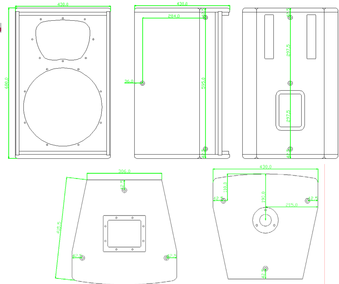
尺寸图 Drawing
